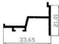
CLIP
