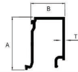
CLIP
