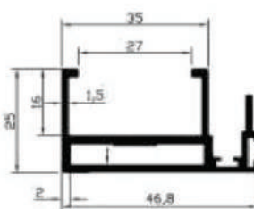
SLIM INTERLOCK DGU
