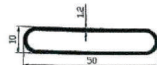
LOUVER BLADE
