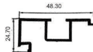
LOUVER CLIP
